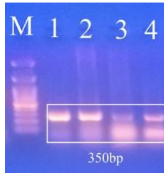
شکل ۵- نتایج آزمون زنجیره‌ای پلی‌مراز معکوس در ژل آگارز ۱٪ شامل نمونه‌های آلوده به پوتی‌ویروس‌ها از گیاه دیفن باخیا. Figure 5- The results of RT-PCR test in 1% agarose gel including samples infected with Potyvirus from Dieffenbachia sp. Plants.
