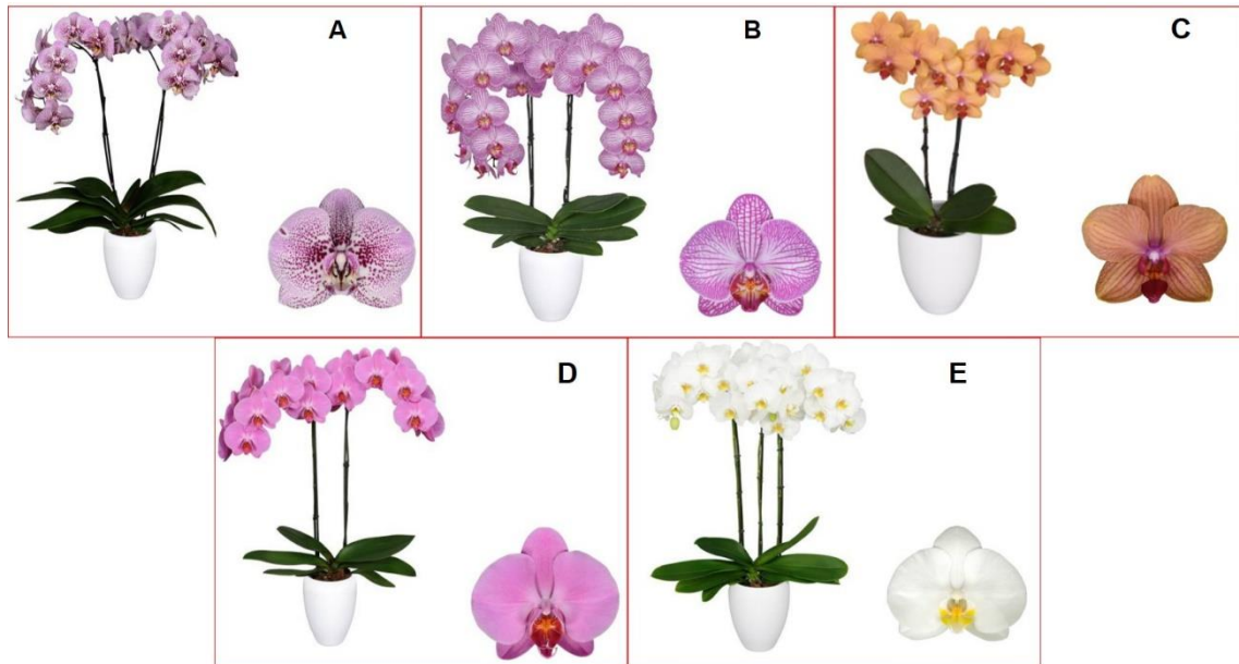
شکل ۱- رقم‌های ارکید فالا‌نوپسیس که در این پژوهش مورد بررسی قرار گرفتند: (A) Andorra، (B) Bucharest، (C) Dubrovnik، (D) Memphis، (E) Nottingham.
