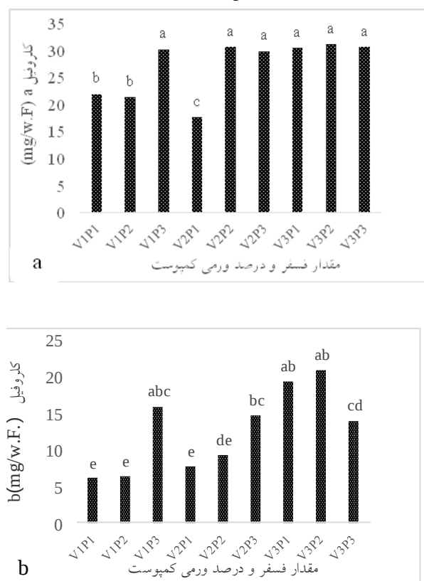
شکل ۶- میزان کلروفیل (a) و کلروفیل (b) آهار تحت تاثیر تیمار فسفر در بستر ورمی کمپوست
