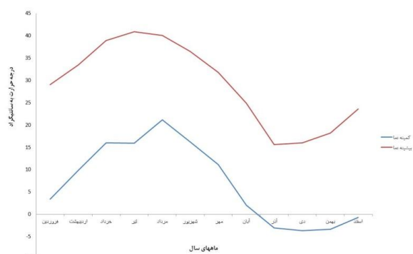
شکل ۳- میانگین دما (۱۳۷۲-۱۳۹۳)
