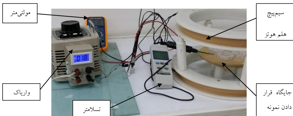
شکل ۱- سامانه اعمال میدان مغناطیس متناوب به بذر چمن
