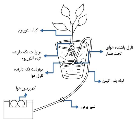
شکل ۲- قسمتهای مختلف سیستم ابروپونیک مورد استفاده (Jowkar 2006)
