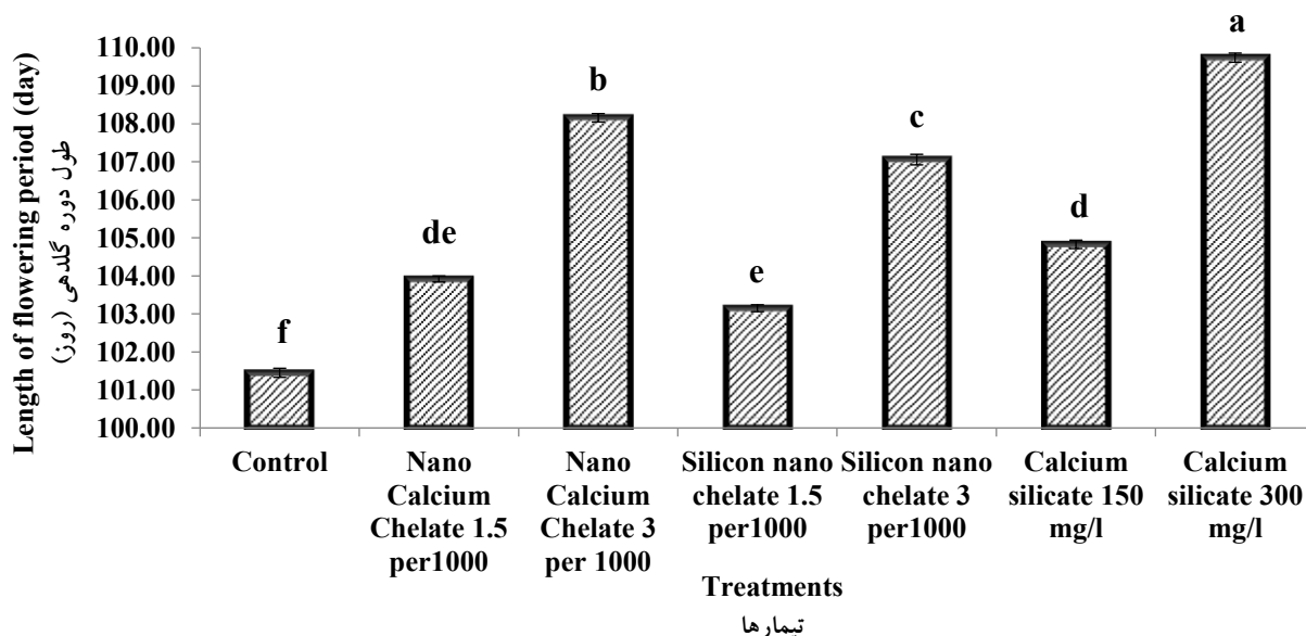
شکل ۷- اثر ترکیبات مختلف سیلیسیم و کلسیم بر طول دوره گلدهی آهار ( Zinnia elegans L.). میانگین‌ها دارای حروف مشابه، بر اساس آزمون چند دامنه‌ای دانکن و در سطح احتمال پنج درصد، تفاوت معنی‌داری با یکدیگر ندارند. (میانگین \pm SD).
