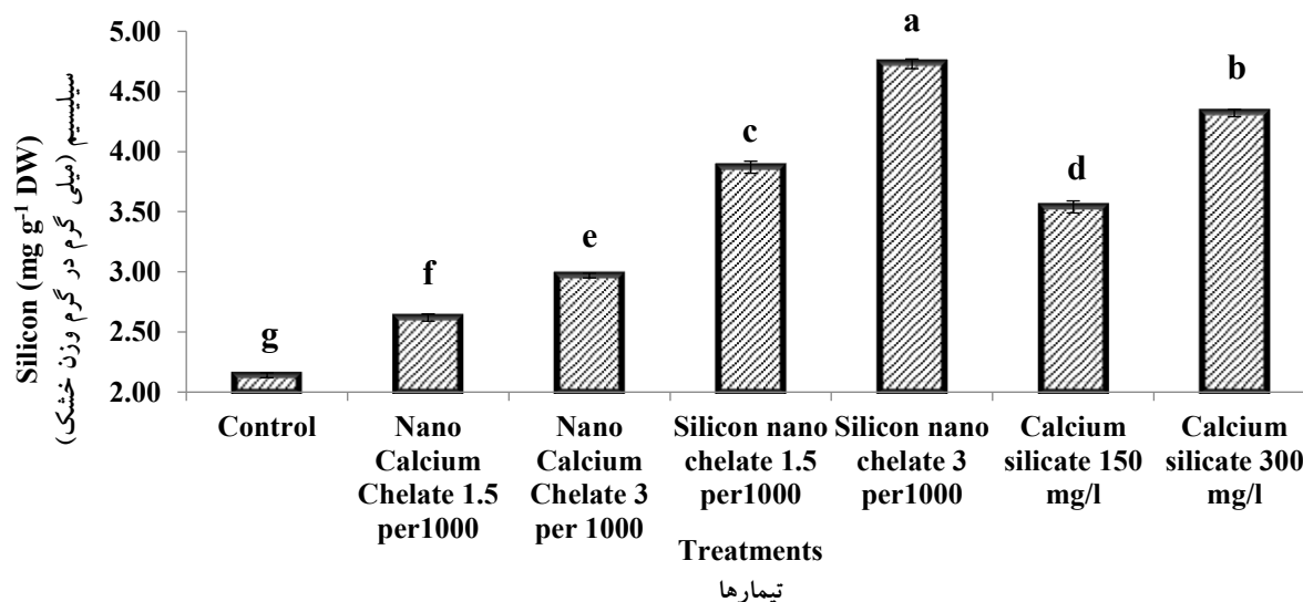
شکل ۵- اثر ترکیبات مختلف سیلیسیم و کلسیم بر سیلیسیم برگ آهار ( Zinnia elegans L.). میانگین‌ها دارای حروف مشابه، بر اساس آزمون چند دامنه‌ای دانکن و در سطح احتمال پنج درصد، تفاوت معنی‌داری با یکدیگر ندارند. (میانگین \pm SD).
