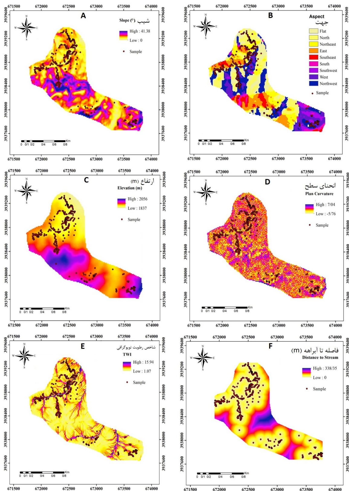
شکل ۲- نقشه‌های شاخص‌های پستی-بلندی ناحیه مورد بررسی؛ شیب (A)، جهت (B)، ارتفاع (C)، انحناى سطح (D)، شاخص رطوبت توپوگرافی (E)، فاصله تا آبراهه (F).
