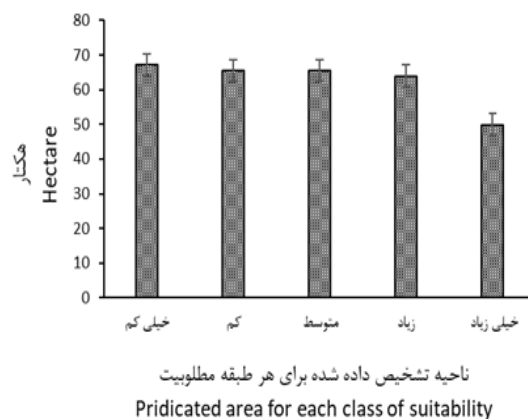
شکل ۹- ناحیه دارای مطلوبیت در هر یک از طبقه‌های تشخیص داده شده توسط MaxEnt.
