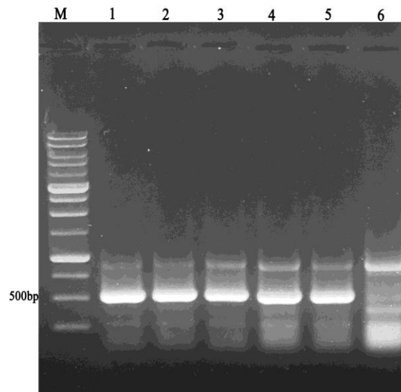
شکل ۲- نقوش الکتروفورزی محصولات RT-PCR تکثیر شده با استفاده از جفت آغازگر عمومی (CarmoIIF/CarmVIR) تیره Tombusviridae روی ژل آگارز ۱٪. M: GenRuler™ 1 kb DNA ladder (Fermentas)، راهک‌های ۵-۱: به ترتیب جدایه های P19، P108، P111 و P112، راهک ۶: شاهد منفی.
