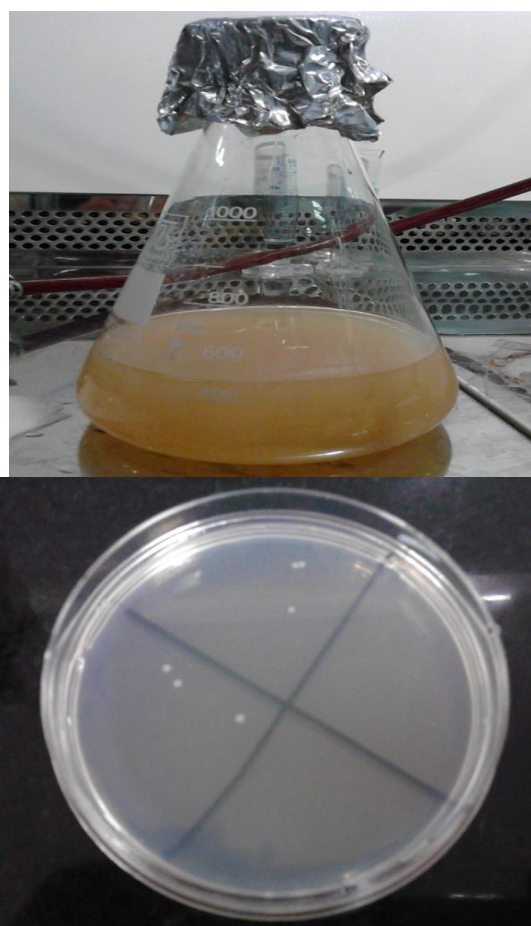
شکل ۶- محیط کشت باکتری (بالا) و تعداد کلونی باکتری در تیمار ۰/۷۵ میلی‌مولار اسید سالیسیلیک (پایین)
