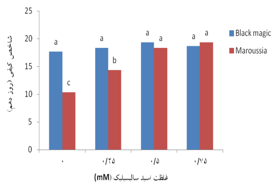
شکل ۳- مقایسه اثر غلظت‌های مختلف اسید سالیسیلیک بر
