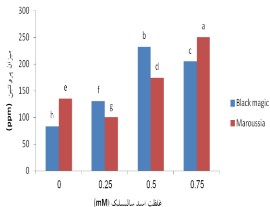
شکل ۱۱- مقایسه اثر غلظت‌های مختلف اسید سالیسیلیک بر میزان پروتئین در دو رقم بلک مجیک و ماروسیا
