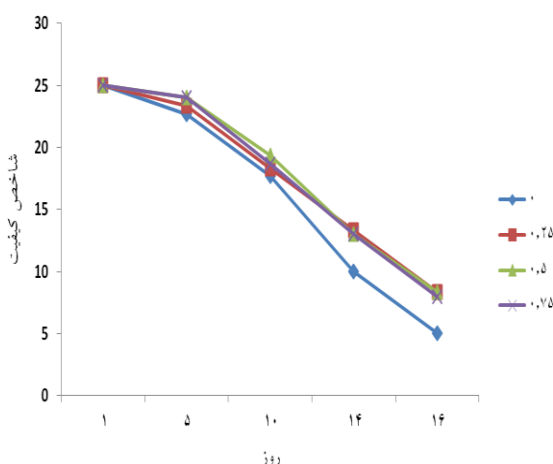
الف) بلک مجیک
