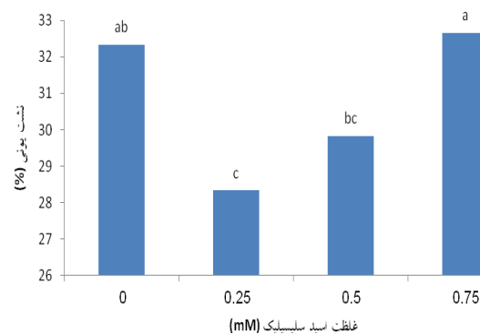
شکل ۲- اثر غلظت‌های مختلف اسید سالیسیلیک بر میزان نشت یونی در رز
