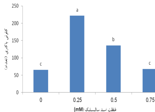
شکل ۷- اثر غلظت‌های مختلف اسید سالیسیلیک بر تعداد کلونی تشکیل شده باکتری در محلول نگهدارنده رز
